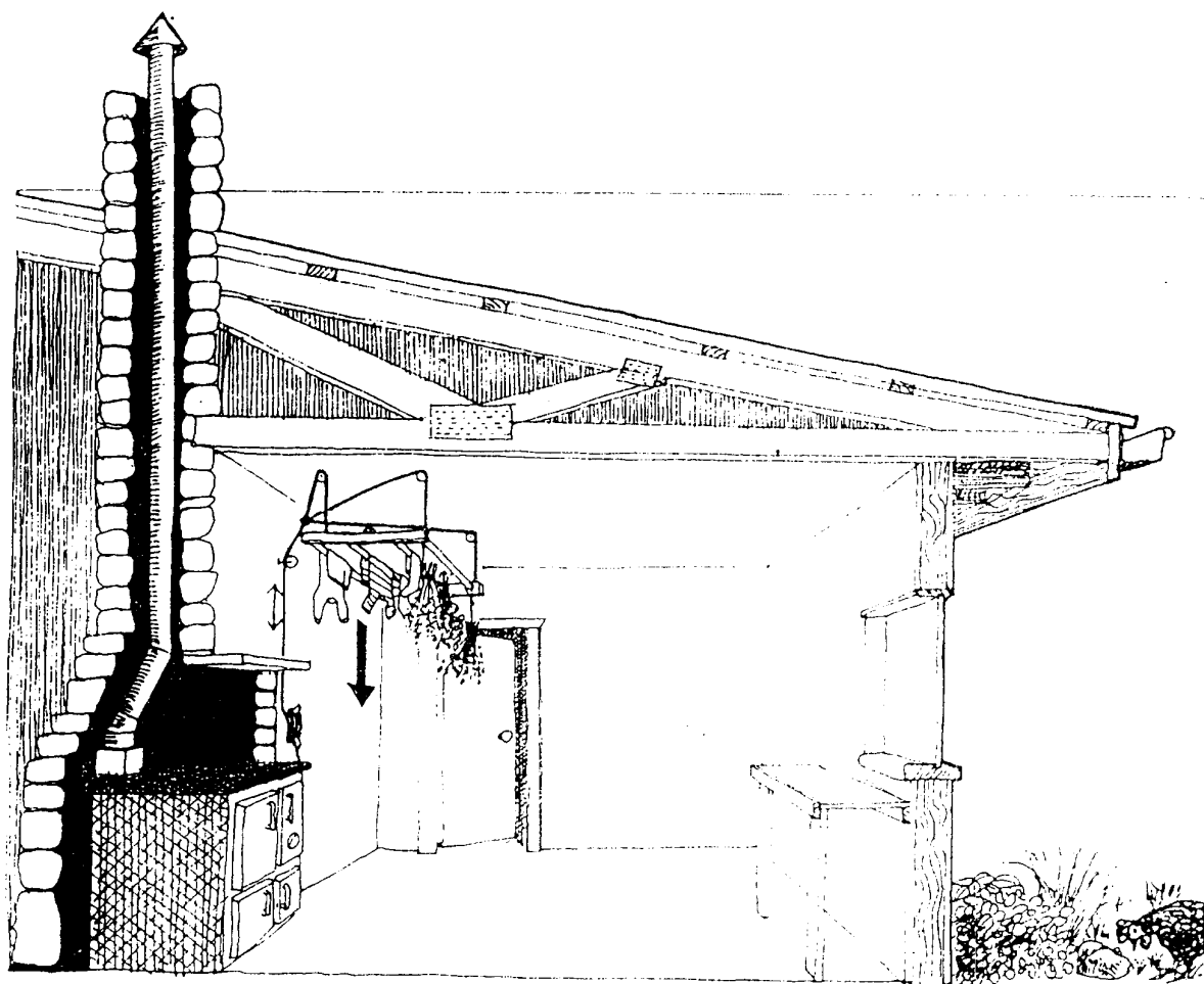
FIGURA 3.24 El sistema de polea para rejilla de secado ubicado sobre la estufa de leña, seca la ropa en el tiempo frío y húmedo.
