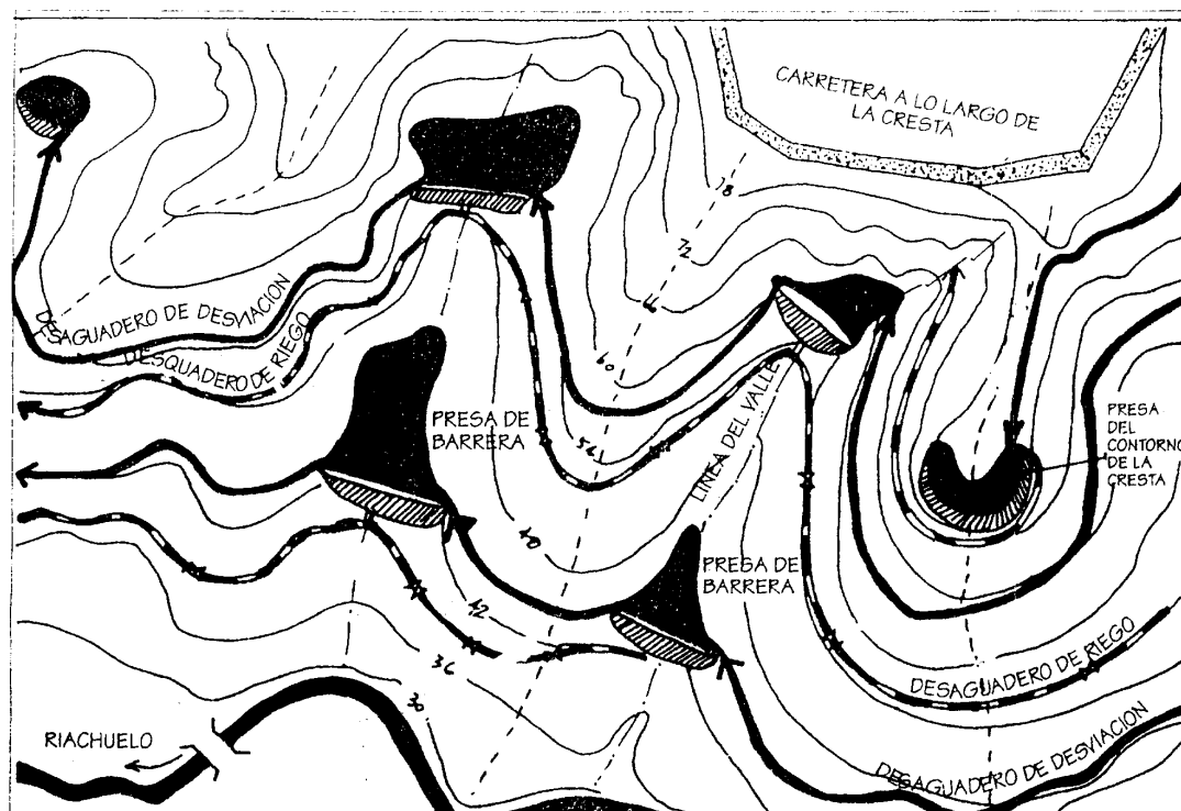
FIGURA 2.27 El sistema de "Línea Clave" de P.A. Yeomans es a prueba de sequía; y funciona en fincas con costos de operación y mantenimiento bajos; su libro incluye diseño total para agua en fincas ubicadas en la base de la colina, accesos, cinturones de árboles, creación de suelos, baja labranza y almacenamiento creativo de agua.
