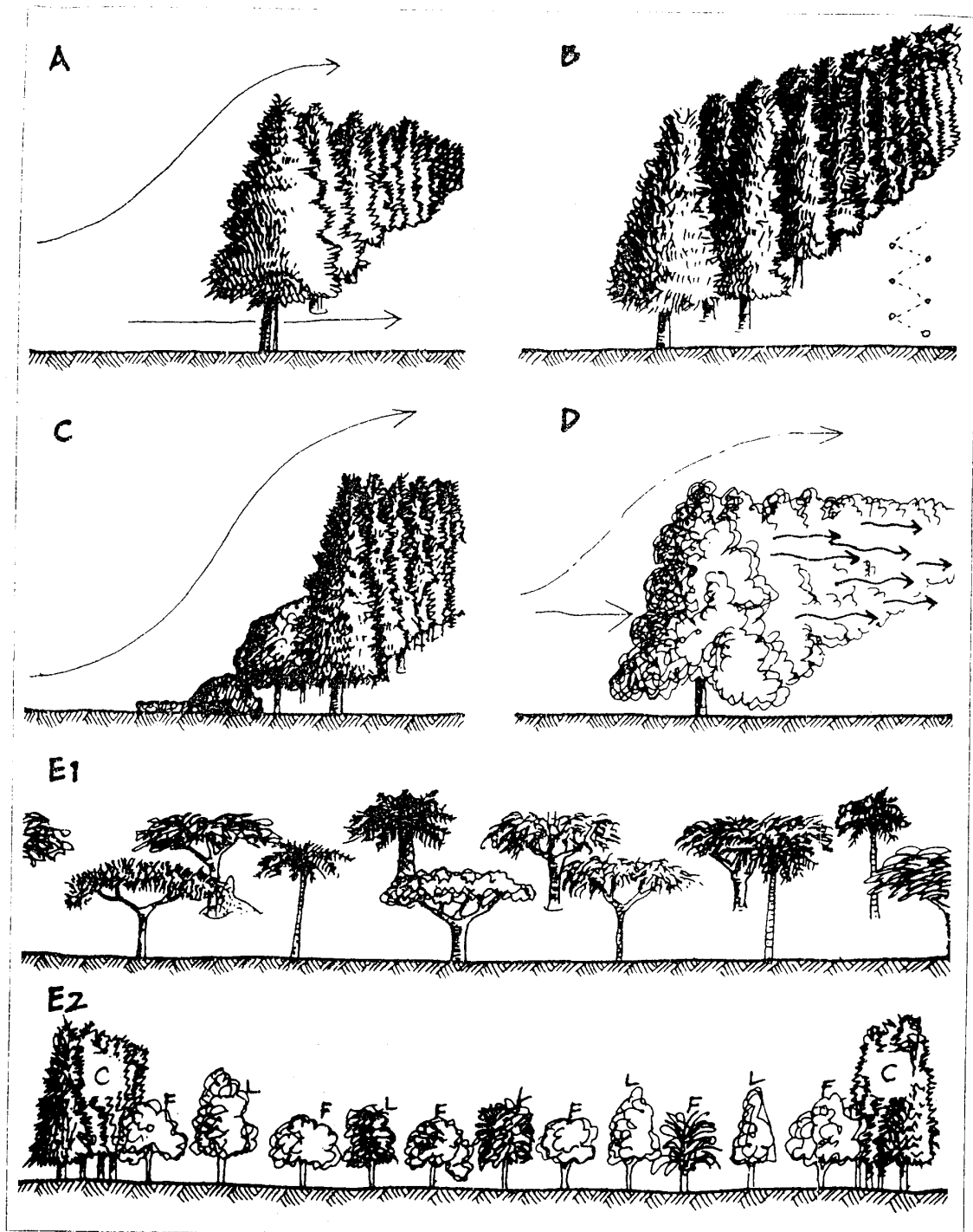
FIGURA 2.15 Configuraciones de rompevientos. No existe el "mejor" rompeviento; cada cultivo, sitio o condición necesita un diseño específico. Aquí (A) para crestas (B) viñas altos (C) la costa (D) campiñas (E 1 ) Cultivos del desierto (E 2 ) Huertos frutales templados. (L=leguminosa, F=árbol frutal, C=conífera o rompeviento).
