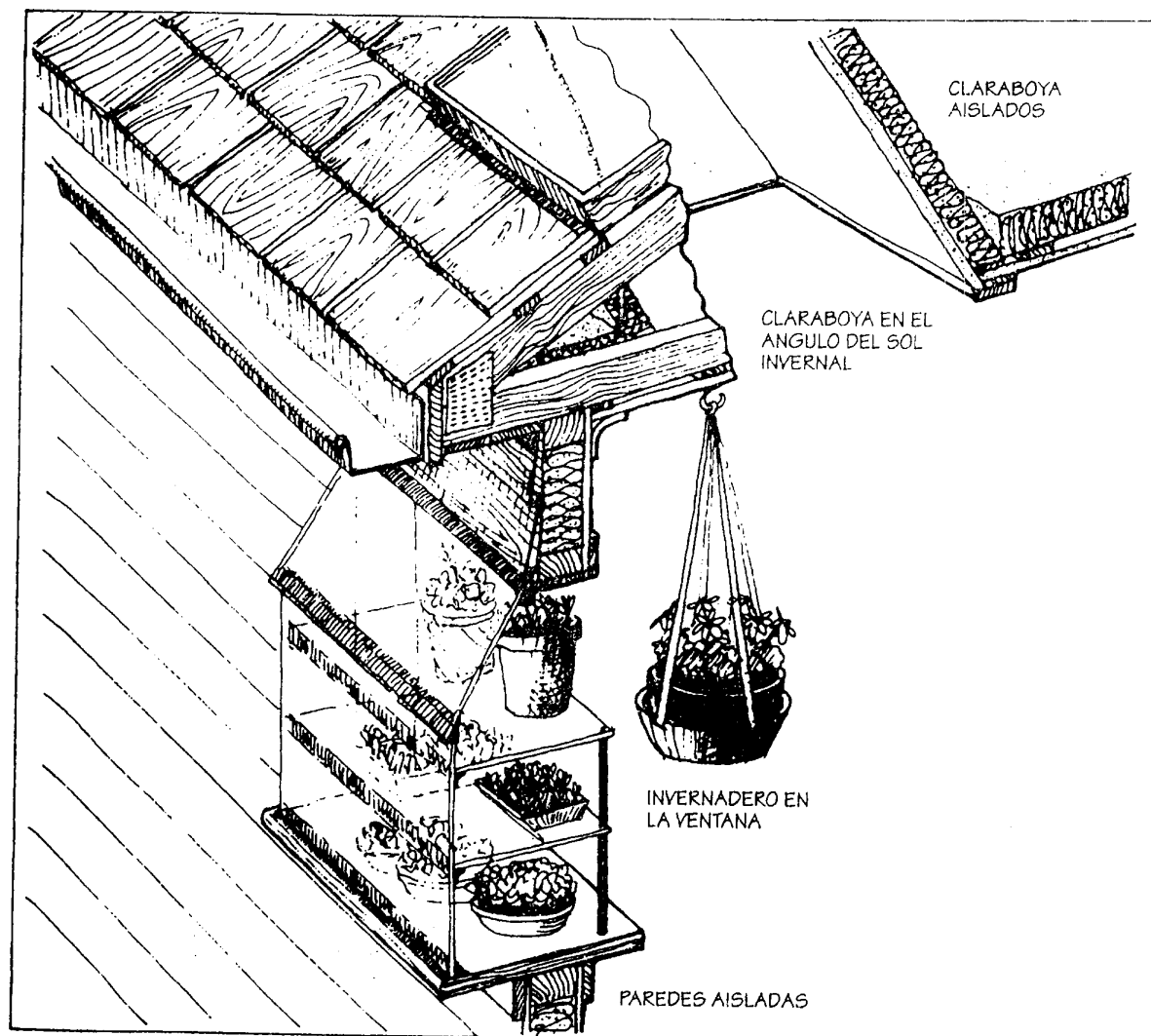
FIGURA 3.10 Invernadero anexo a una ventana y claraboya. Note el aislamiento para retener calor e impedir el frío.
