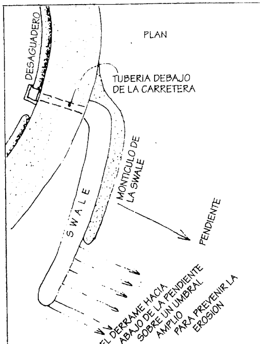
FIGURA 2.30 El agua procedente de las carreteras de la colina llega a un tubo ubicado bajo la carretera y luego pasa a los swales para evitar la erosión del suelo.
