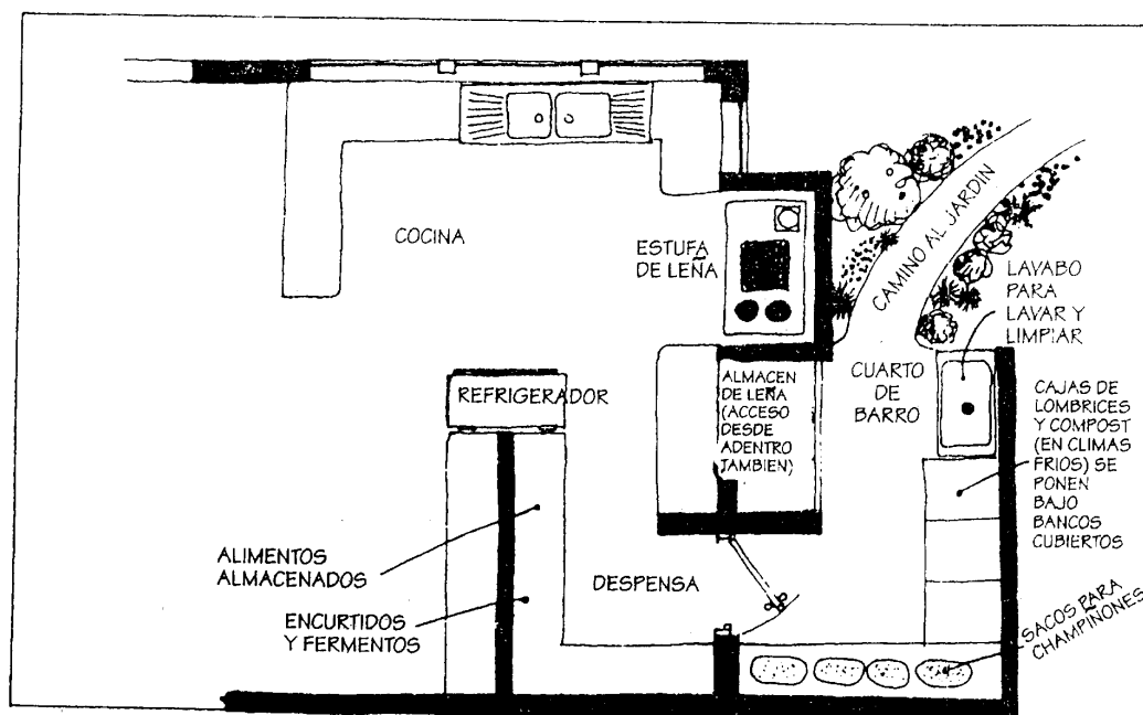
FIGURA 3.4 El "cuarto de lodo" como un área de preparación y almacenamiento, une el jardín a la cocina.
