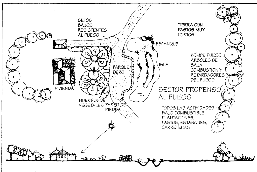
FIGURA 2.31 Diseño combinado para seguridad contra el fuego: escudos de radiación, rompefuegos múltiples abajo de la colina multiple, plantas "húmedas" selectas y reducción de combustibles cerca de la casa.
