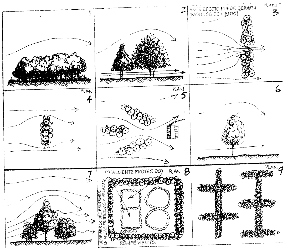
FIGURA 2.16 ROMPEVIENTOS INEFECTIVOS: (1) Muy amplio (2) corte de las ramas bajas, ramaneo o corte por muerte: aceleración de viento (3) velocidad en los claros (efecto de Venturi) (4) muy corto (5) no ubicada perpendicular a los vientos (6) solo una línea de árboles. ROMPEVIENTOS EFECTIVOS (7) líneas de árboles pequeños, medianos y grandes con aproximadamente 50% de permeabilidad para un flujo de aire mejor (8) combinación de rompevientos y seto para tener una protección total donde sea apropiado (vientos costeros, vientos áridos secos desecantes). No apropiados en áreas propensas a heladas a menos que los rompevientos se abran para la liberación del flujo de aire frío. (9) Rompeviento en forma de "T" para el flujo regular de aire y protección.
