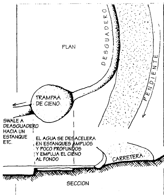
FIGURA 2.29 El agua de escorrentía de la carretera llega a una trampa de cieno, este es sacado de la trampa periódicamente para tierra de macetas.
