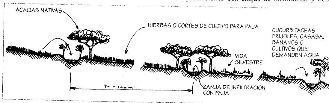
FIGURA 2.22 La distancia entre las zanjas de infiltración en tierras áridas es mayor que en los climas húmedos. Las zanjas de infiltración sobre pendientes sirven para cultivar legumbres para pienso y árboles resistentes. El espacio entre las zanjas puede sembrarse con hierbas o granos después de las lluvias sobre suelos arados.
