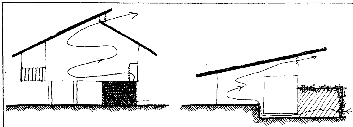
FIGURA 3.12 Techos con rejillas de ventilación permiten que el aire caliente del cuarto escape y los enrejados permiten que el aire frío entre.
