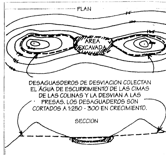
FIGURA 2.24 Las presas son útiles para el control de fuego, la vida silvestre, el riego limitado. Este es el tipo de presa más alto en el paisaje que se llena con la escorrentía de la colina.
