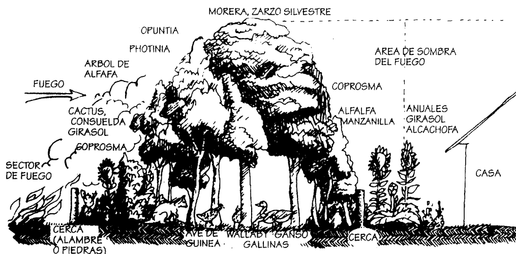
FIGURA 2.32 Plantación contra el fuego (con ganado) para pueblos pequeños o sitios con casas.
