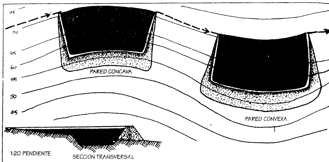
FIGURA 2.28 Las presas de contorno son prácticas en pendientes de 8° o menos, como parte de una serie general de presas en la granja.
