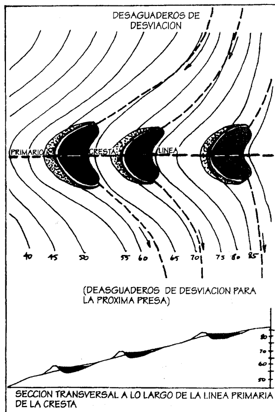
FIGURA 2.25 Las presas en los puntos de crestas de montaña se construyen sobre las áreas planas (aplanadas) de las crestas.
