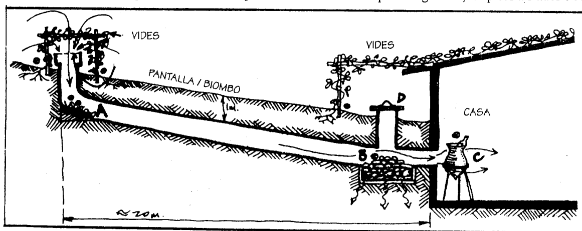
FIGURA 3.15 El túnel de tierra provee aire fresco húmedo a las casas de los desiertos. La pendiente del túnel baja hacia la casa, es sombreado en su abertura al exterior, tiene una cama húmeda compuesta de ceniza gruesa(B) y una vasija (no de vidrio) con agua en la salida del aire. Su longitud es de 20 metros.
