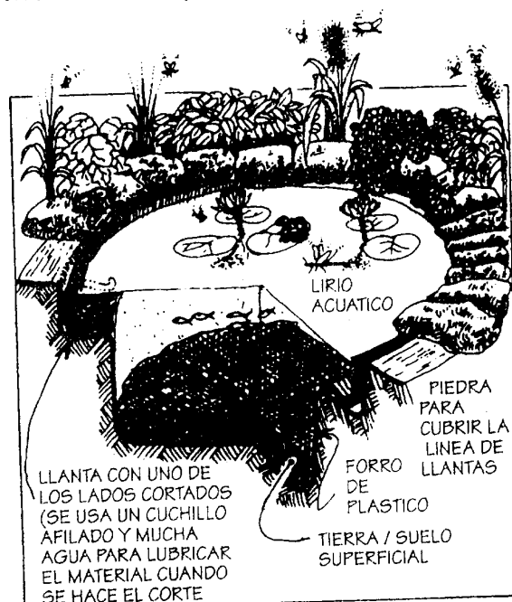
FIGURA 4.9 Jardín de estanque de llantas con lirios acuáticos, plantas de borde, ranas, insectos y peces.
