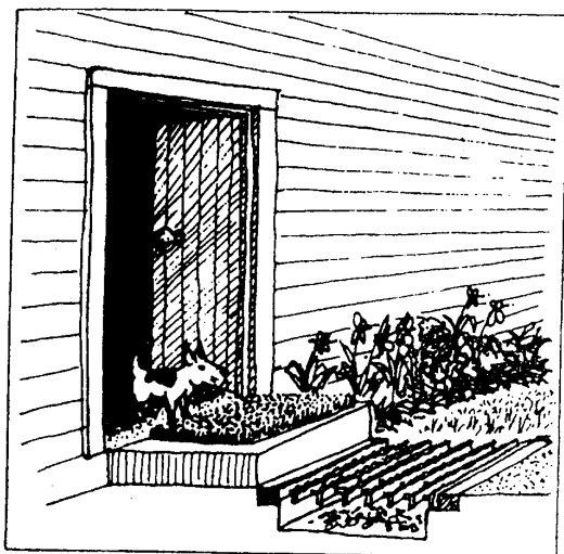
FIGURA 3.3 Parilla y felpudo para remover el lodo de las botas en la entrada de la casa.
