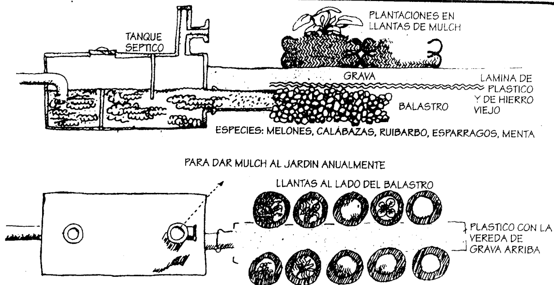
FIGURA 3.22 Disposición del contenido de un tanque séptico a través de una línea de llantas con plantas.
