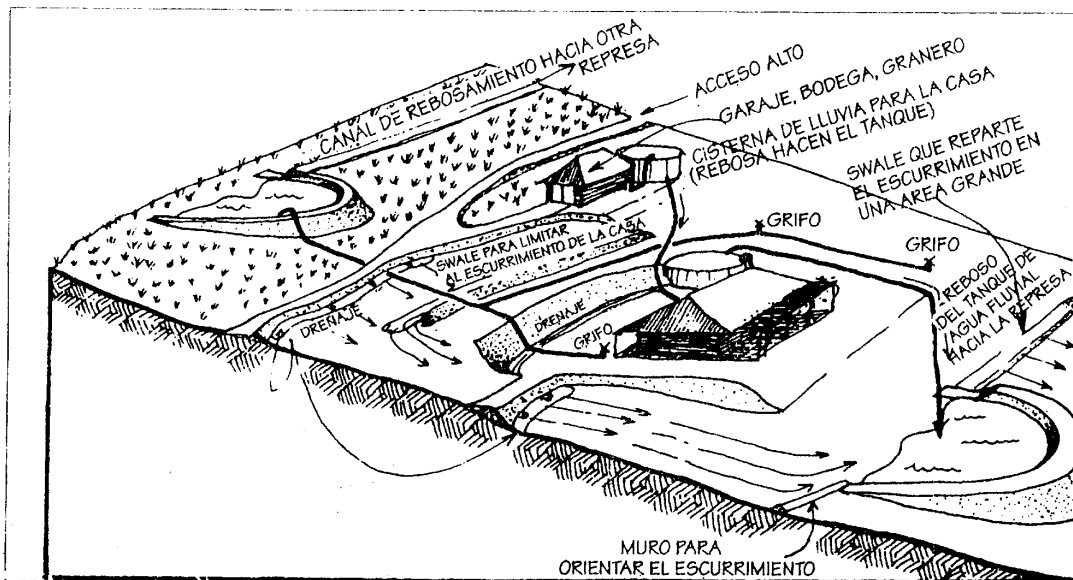
FIGURA 1.7 Representación ideal de la ubicación del agua, los edificios, y el acceso (no se indica la vegetación a fin de demostrar mejor el movimiento de agua). Las zanjitas distribuyen el agua sobre una pendiente ancha donde existe yerba, a fin de evitar la erosión hidráulica durante las temporadas lluviosas.
