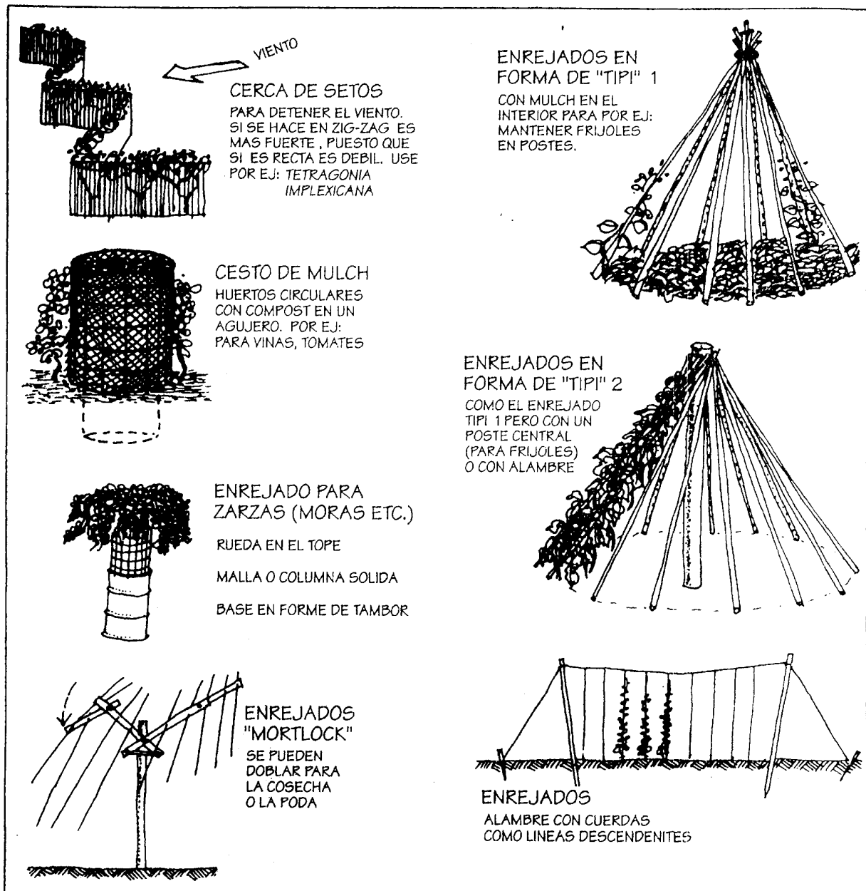
FIGURA 4.7 Los sistemas de enrejados en el campo o en el huerto amplían grandemente el espacio de cultivo.
