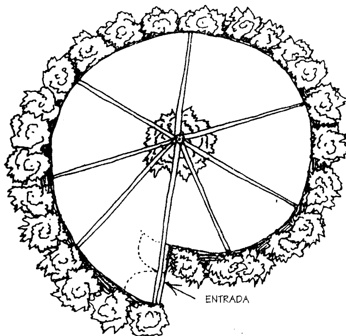
FIGURA 3.20 Abrigo económico para animales domésticos mayores: Plano (A) vista desde arriba y (B) abajo. El piso es de lozas o de concreto y las paredes son una espiral de bambú o álamo, con un centro formado por un árbol ya existente o un poste. Las paredes son entretejidas y cubiertas por hiedra que va hasta el techo.
