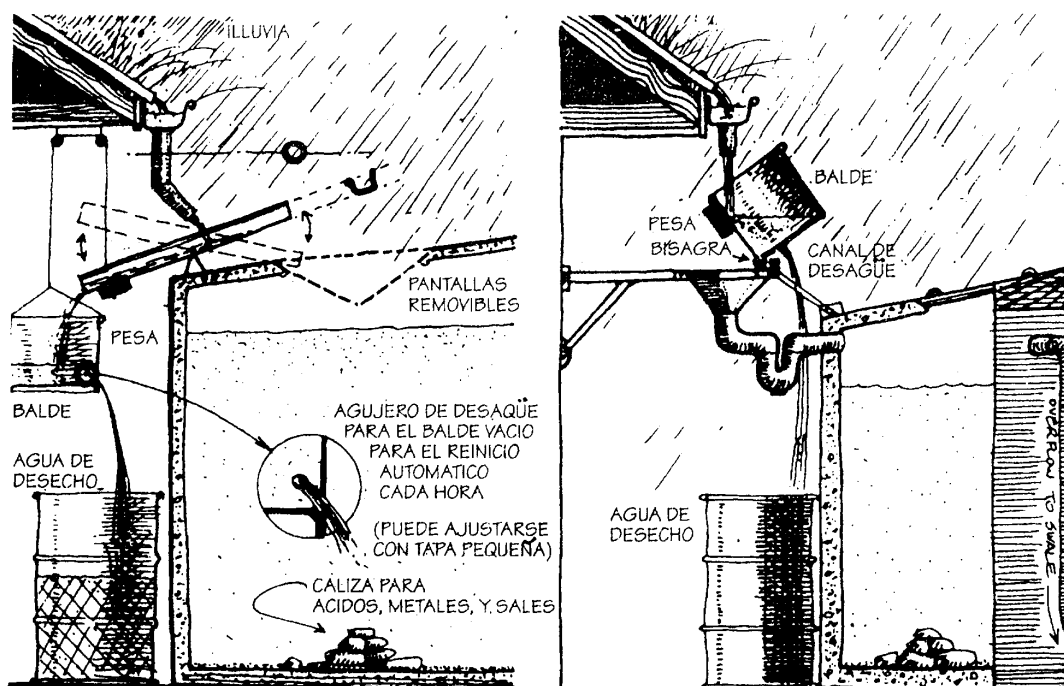
FIGURA 2.23 Dos maneras para expulsar el primer flujo de agua de un techo (para polvo y desechos de hojas). Ambos sistemas vuelven automáticamente a su posición original cuando vacíos.
