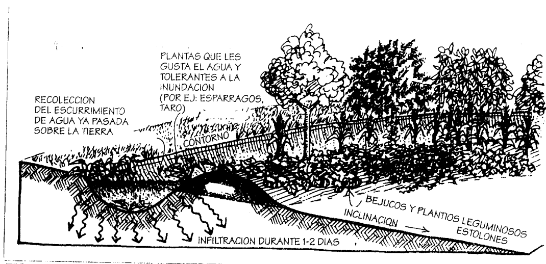
FIGURA 2.21 Zanjas de infiltración sobre el contorno no fluyen; ellas primero paran y luego absorben el flujo de agua que está sobre el suelo. Las zanjas de infiltración se plantan con árboles o arbustos sobre el lado del montículo.
