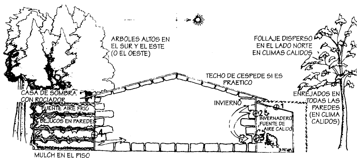
FIGURA 3.9 El aire frío circula desde la casa de sombra hasta la casa, atraído a ésta desde el invernadero. Los bejucos deciduos (vides) están ubicados en el lado soleado, mientras que los bejucos siempre verdes están en el lado sombreado.
