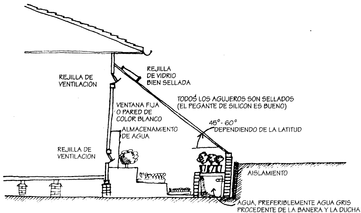
FIGURA 3.8 Un invernadero en el lado soleado de la casa puede ayudar en la calefacción, especialmente en los climas de inviernos fríos. Las rejillas de ventilación son esenciales para brindar calor al interior de la casa durante el invierno y el verano fresco.
