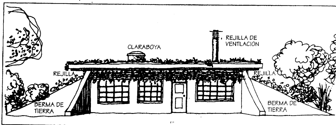
FIGURA 3.18 Las casas de terraplenos apisonados en los climas áridos mantienen la casa aislada y fresca. Los bejucos pueden sombrear las paredes que miran al sol.
