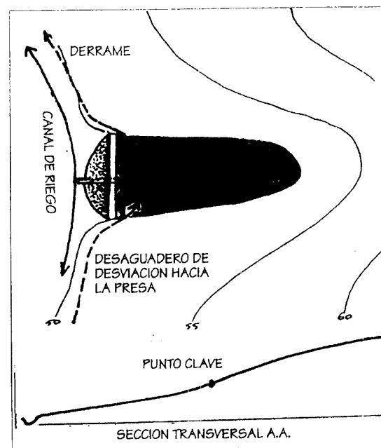
FIGURA 2.26 Presa de punto clave. Si es usada en serie, no ocurre el derrame y el flujo va a la próxima presa, y eventualmente a un riachuelo. Junto a un sistema de riego sirve para pendientes bajas.
