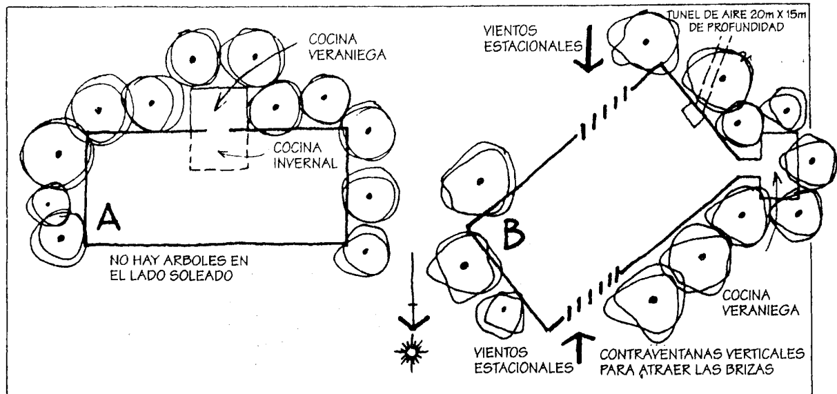
FIGURA 3.11 Ubicación de casas en (A) los subtrópicos, donde la orientación es hacia el sol debido a los inviernos fríos, y (B) los trópicos, donde la orientación es hacia las brisas frescas y la casa está rodeada por la sombra.
