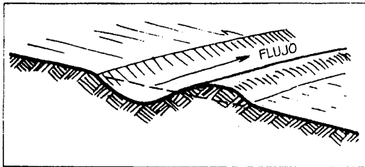
FIGURA 2.19 Desviación del flujo de desagüeros de los riachuelos a las presas o colección del el flujo de agua y llevarlo a las presas. Ellas son una parte vital de cualquier sistema de colección de agua de lluvia.
